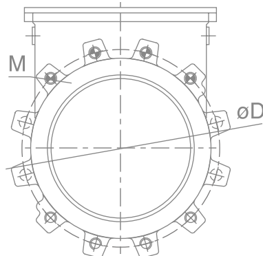
NPS 20-24
