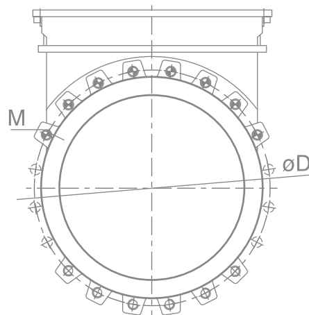
Detalles de bridas y pernos
